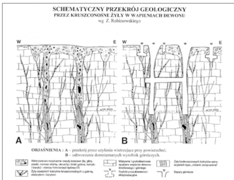
Schemat użyłen i wyrobisk górniczych; rys. Z. Rubinowski
